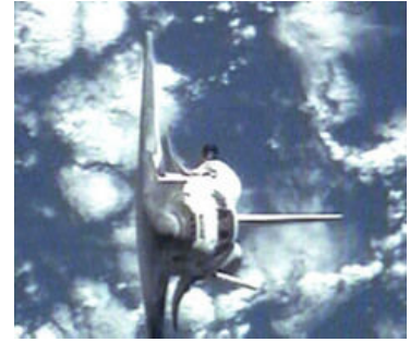
Immagine NASA: il Discovery si allontana dalla Terra
